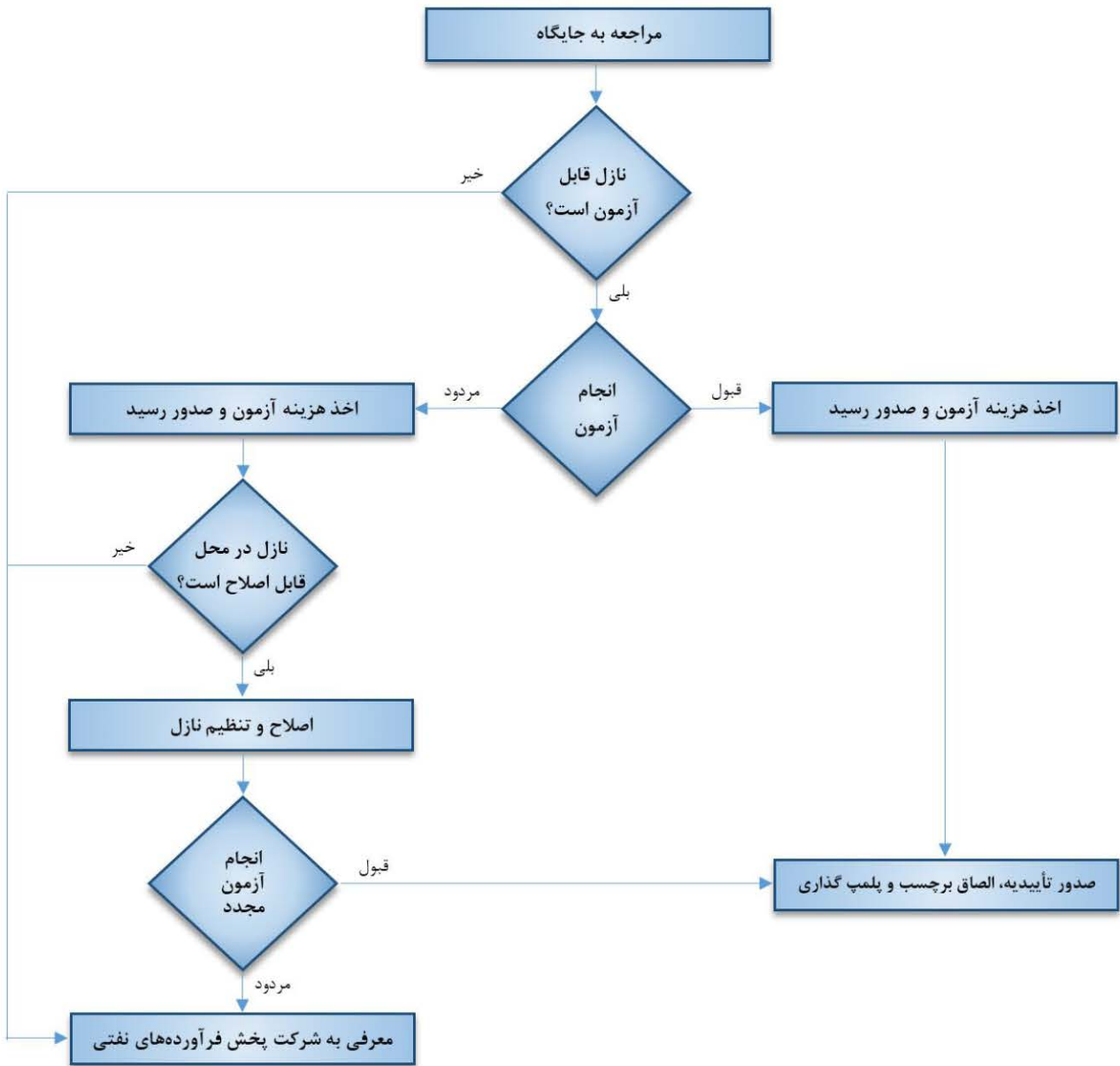
فلوجارت (۲) : فرآیند اجرای آزمون نازل‌های عرضه سوخت مایع
